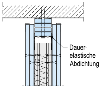
Abb. WK. 2: Gleitender Deckenanschluss einer Metallständerwand
