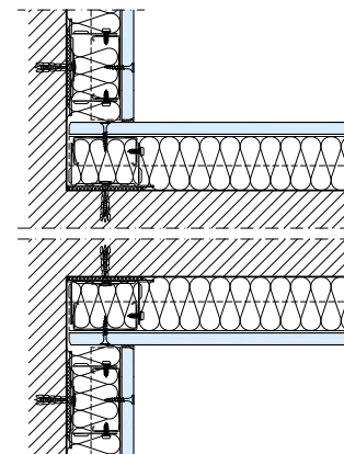
Abb. WK. 4: Vorsatzschale bei Trennwand mit flankierendem Bauteil
