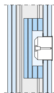
Abb. WD. 1: Umbauen mit Gipsplatten
